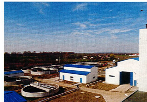
Fig. 8. Modernizarea cu treaptă terțiară a Stației de epurare Satu Mare.
