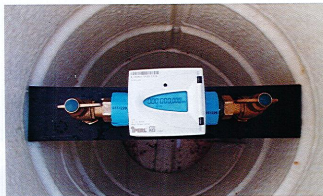
Fig. 10. Contoare cu citire la distanță.
